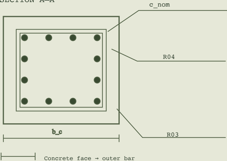
04 / SECTION A-A
